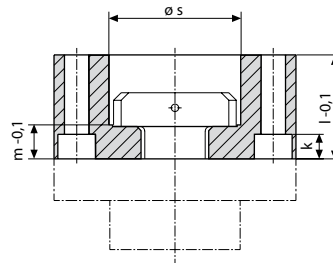
Flange
